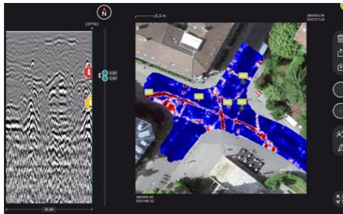
GS9000：使用予定の地下埋設物機材とスキャンデータのマッピングイメージ図
